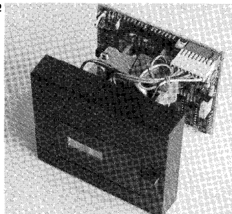
afb. 1 De SERCOS serie interface module.
