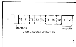
Afb. 1 Voorbeeld van karakteropbouw bij asynchrone seriële transmissie.
