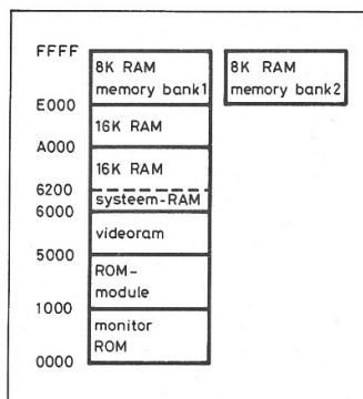
Afb. 1 De geheugenopbouw.
