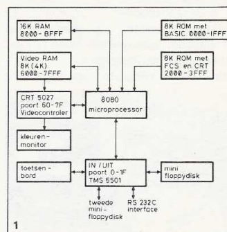
afb. 1 De opbouw van de Compucolor II.
