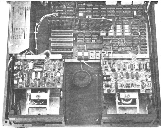
Afb. 2 Blik in de Basis 108. Afb. 3 Achterzijde van de Basis 108 waarbij de handige aansluitingen voor de netvoeding van printer en monitor opvallen.
