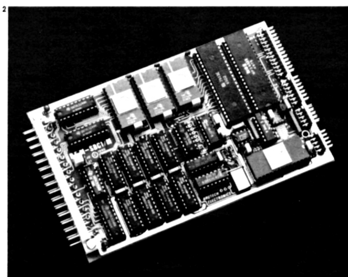
afb. 1 De CPU-2-kaart van het BEM-systeem met als processor de 6809.
