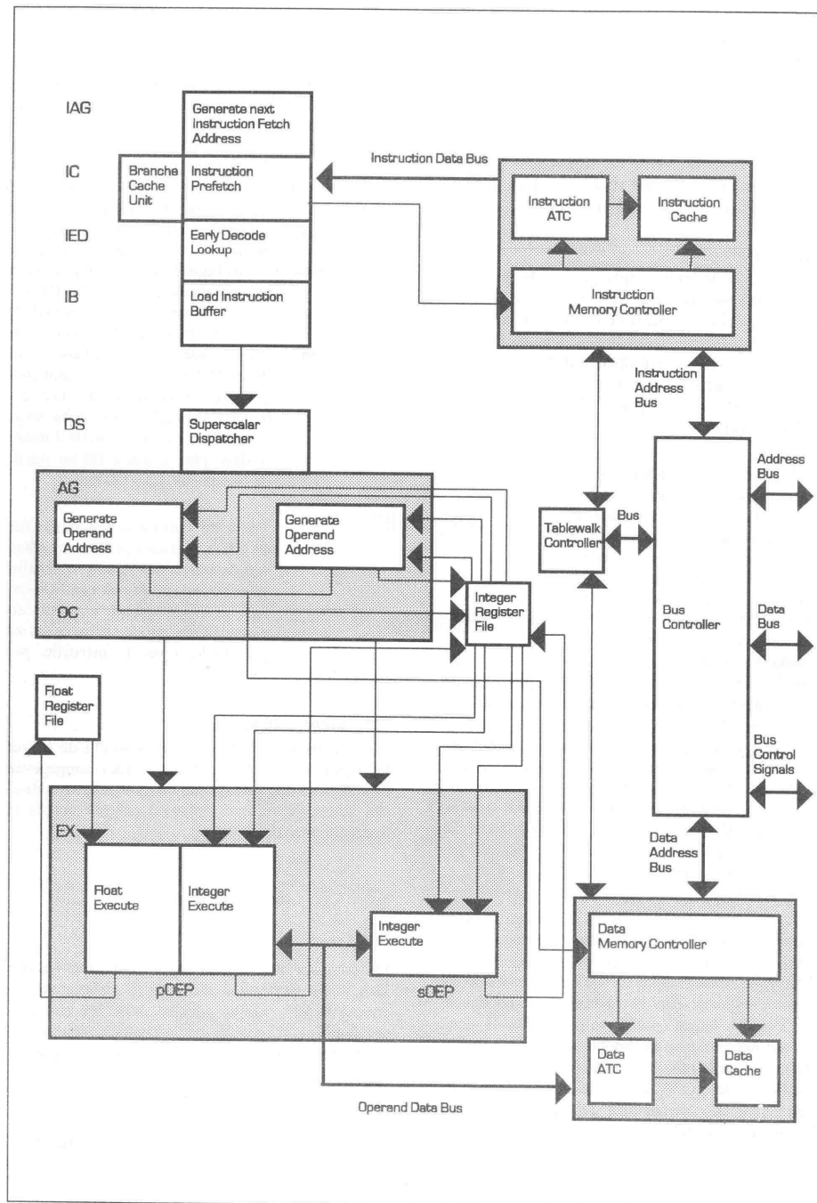
Fig. 1: interne opbouw van de 68060
