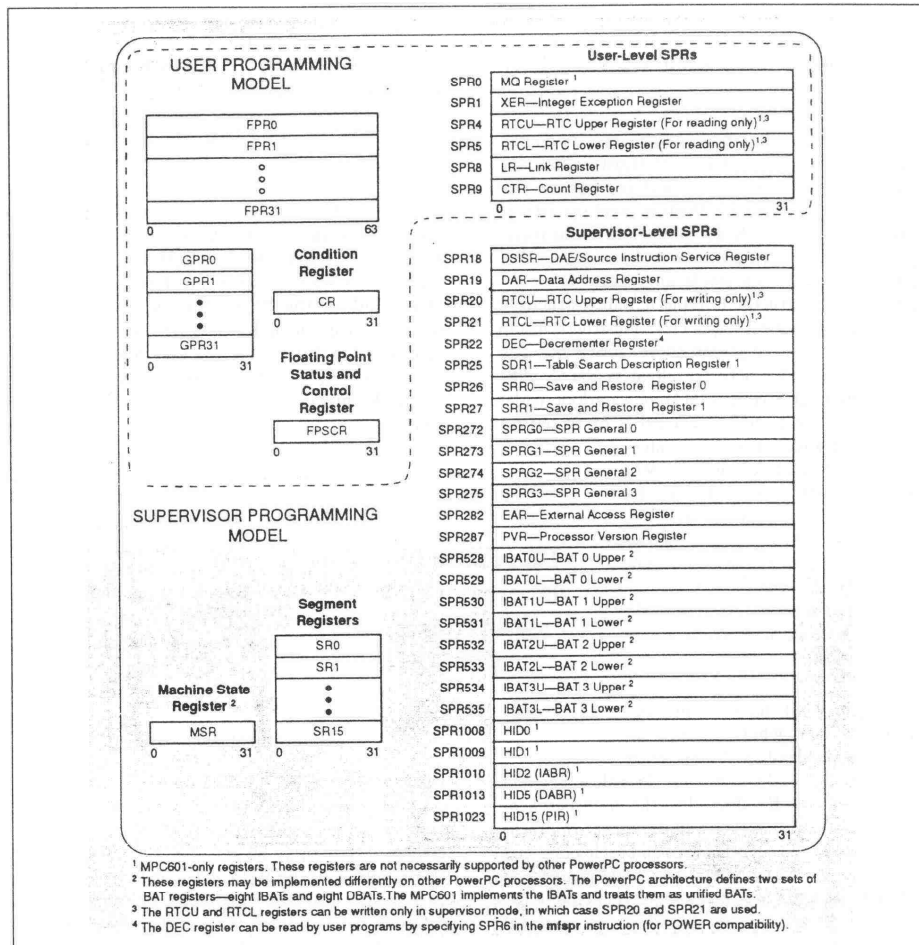
Fig. 1: programmeermodel van de MPC 601 Power PC
