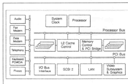
Fig. 3: voorbeeld van een Power PC configuratie
