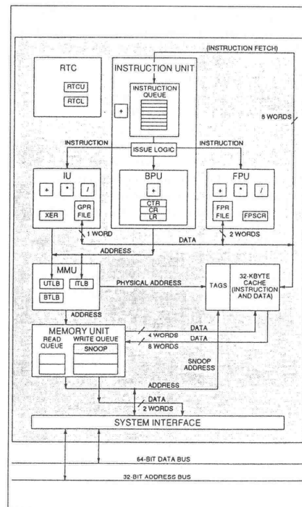
Fig. 1: interne opbouw van de MPC 601 Power PC
