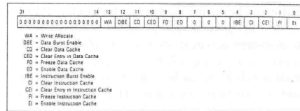
Fig. 4: het cache control register
