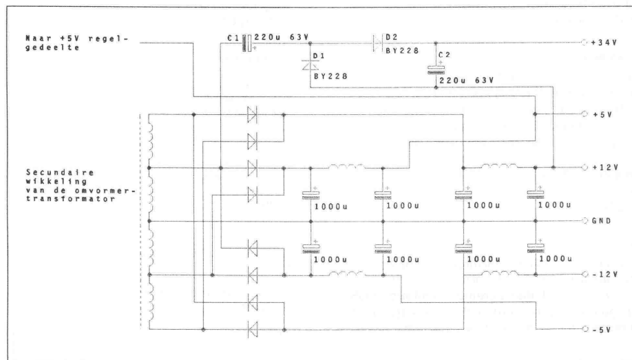
Afb. 1: uitbreiding PC-voeding voor +34 Volt
