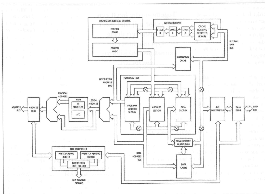
Fig. 1: interne caches van de 68030
