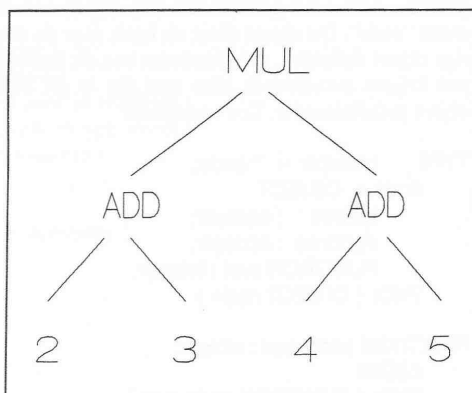
Fig. 1: De parsertree voor (2+3)*(4+5)
