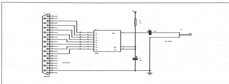
Fig. 1: covox in mono uitvoering
