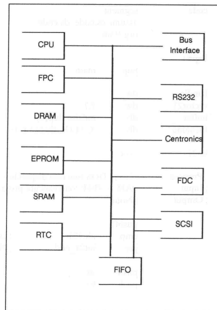
Fig. 1: blokschema van de KGN30
