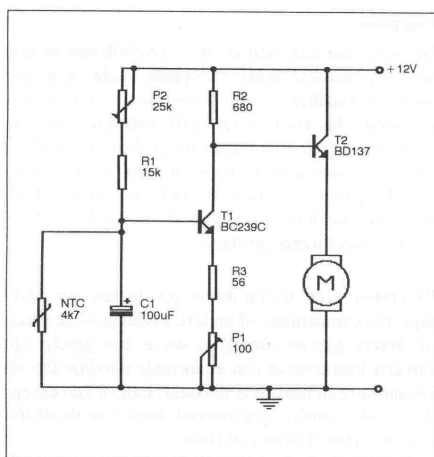
Fig. 1: ventilatordimmer
