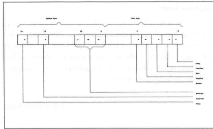
Fig. 2: het statusregister
