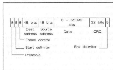
Fig. 3: packet-formaat in een Token Bus protocol
