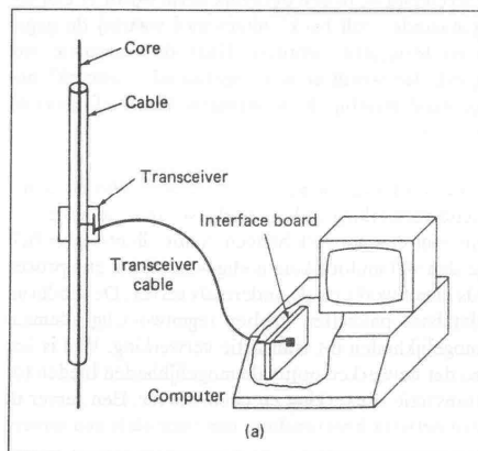
Fig. 1: aansluiting van een computer op een Ethernetkabel
