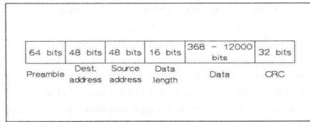
Fig. 2: opbouw van een Ethernetpacket
