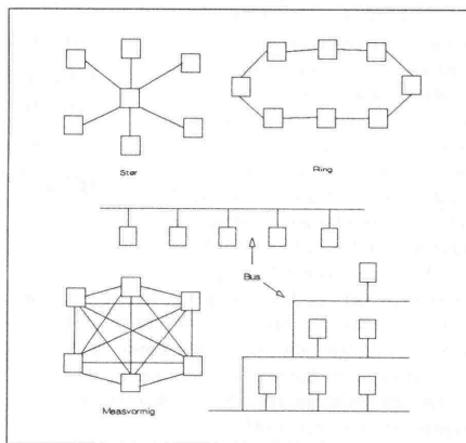
Fig. 1: enkele netwerk-topologieën
