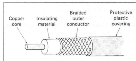
Fig. 3: doorsnede van een coaxkabel
