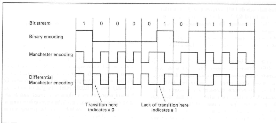
Fig. 5: voorbeelden van het coderen van bits
