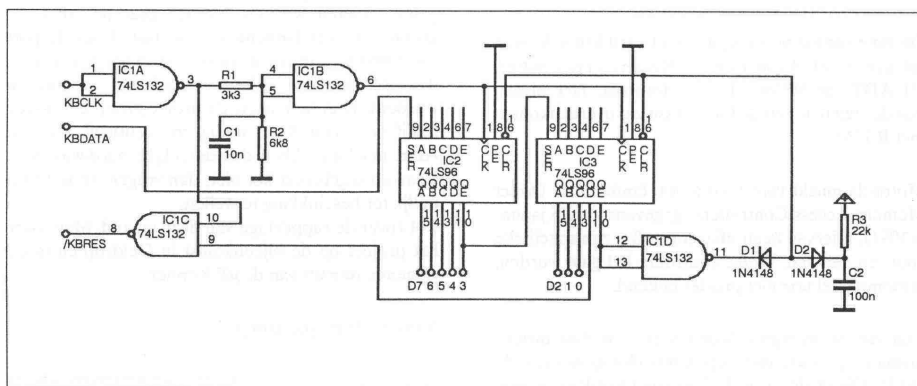
Fig. 1: toetsenbordinterface schakeling
