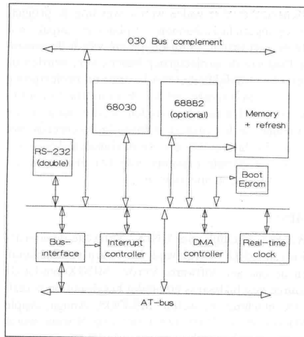
Fig. 1: blokschema van het KGN-68k systeem
