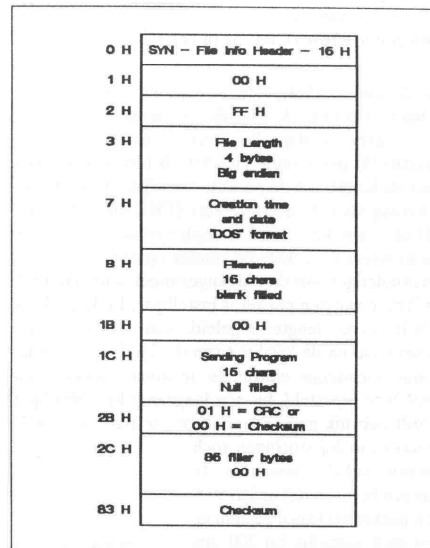
Fig. 2: beschrijvings-packet van het TeLink protocol
