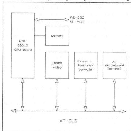
Fig. 1: het KGN-68k bord omringd door AT-hardware
