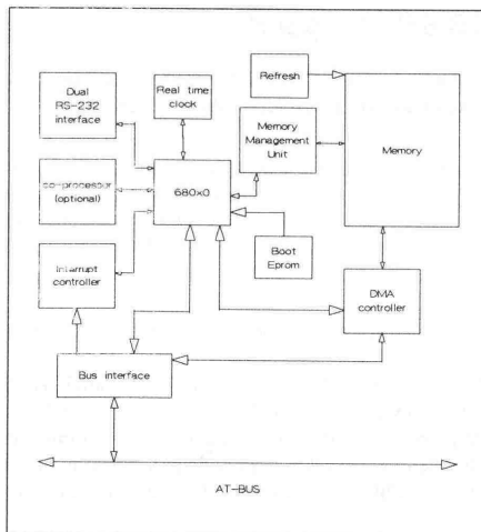
Fig. 2: mogelijk blokschema van het KGN-68k bord
