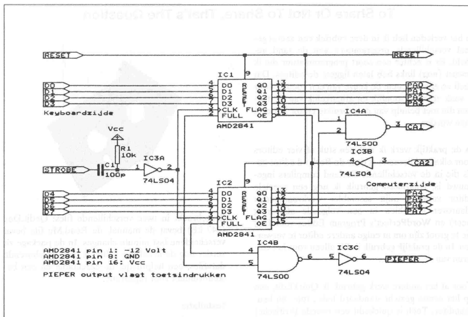
Fig. 2: keyboardbuffer voor DOS65
