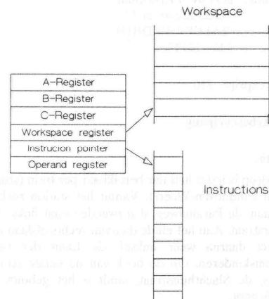
Fig. 5: Werking van work- en instruction pointer
