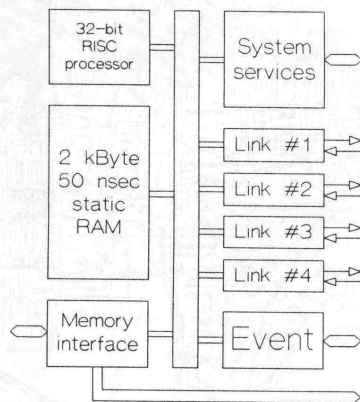
Fig. 4: De T414 van INMOS
