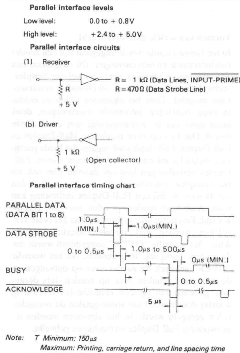
Fig. 2: Signaal-niveaus en timing in de Centronics definitie
