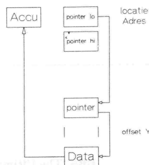
Fig. 7: LDA [ADRES],Y
