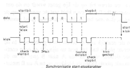
Fig. 3: Tijddiagram voor seriële communicatie
