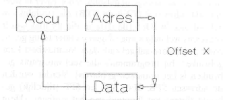
Fig. 1: LDA,X
