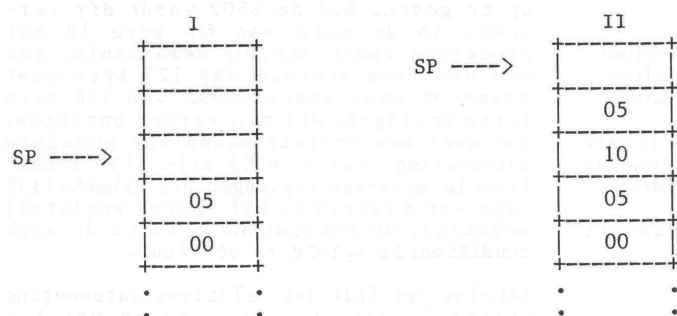
Figuur 6. Voorbeeldprogramma met een geneste subroutine
