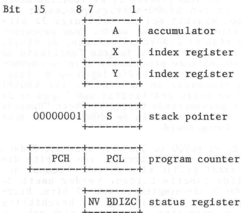
Figuur 1. Programmeermodel 6502.
