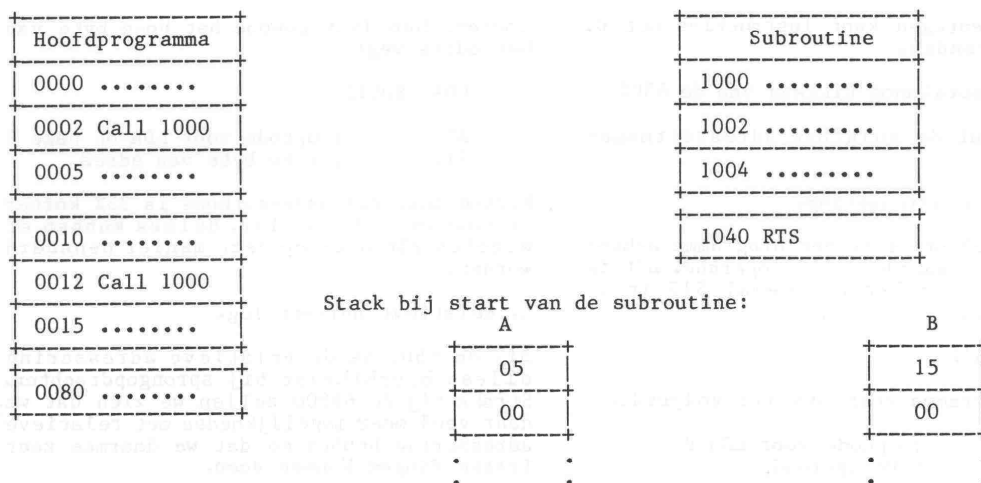
Figuur 5. Voorbeeldprogramma met subroutine
