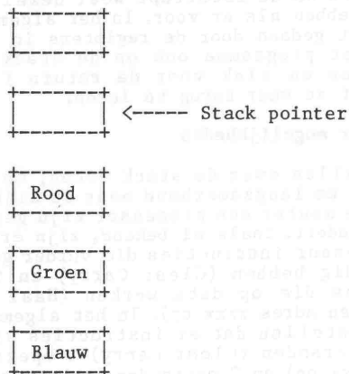
Figuur 4. Voorbeeld van een stack
