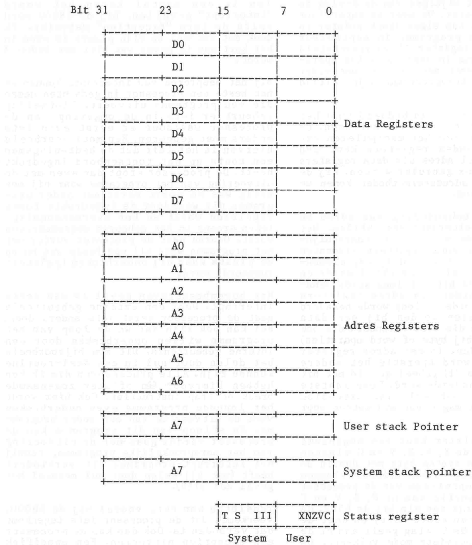
Figuur 3. Programmeermodel 68000.
