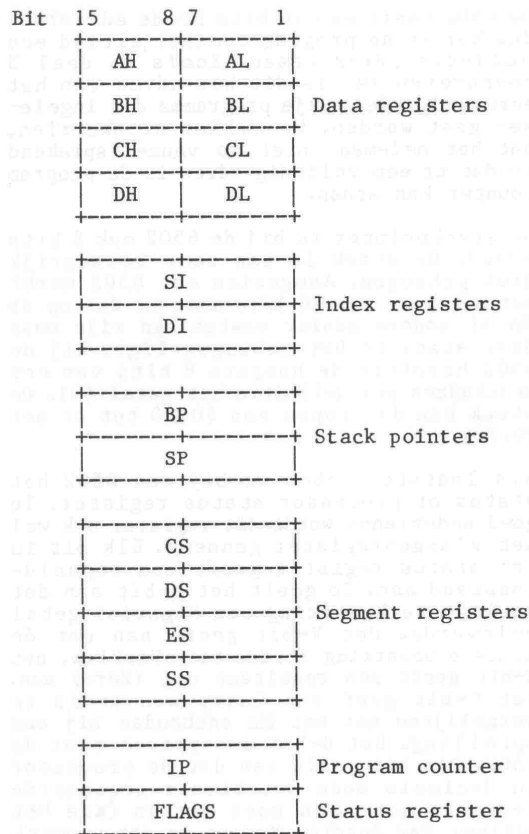
Figuur 2. Programmeermodel 8088.
