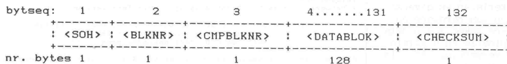
Fig: Xmodem blokformaat. (SOH is altijd $01) Indien Xmodem gebruikt wordt, bestaat de checksum uit twee bytes, te weten CRCHI en CRCLO.
