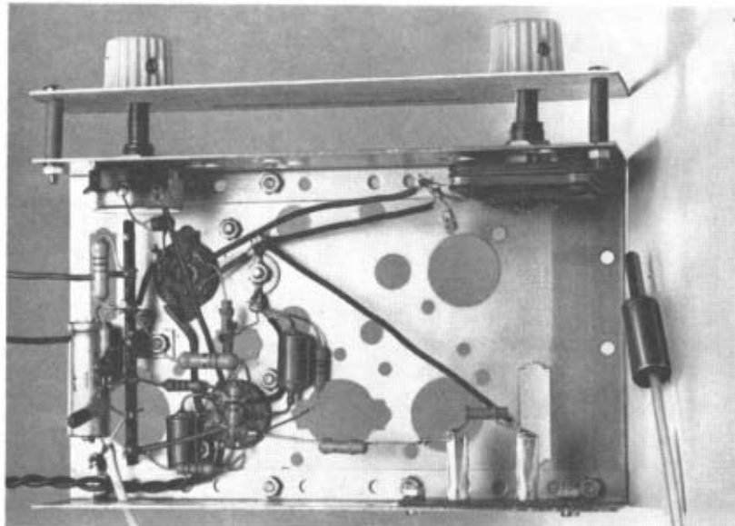
Afb. 12. Overzicht van de bedrading aan de onderzijde van een gebouwde éénkrings-afstemeenheid Pioneer S 101. Controleer ook aan de hand van deze foto de montage, alvorens het toesteltje af te werken.
