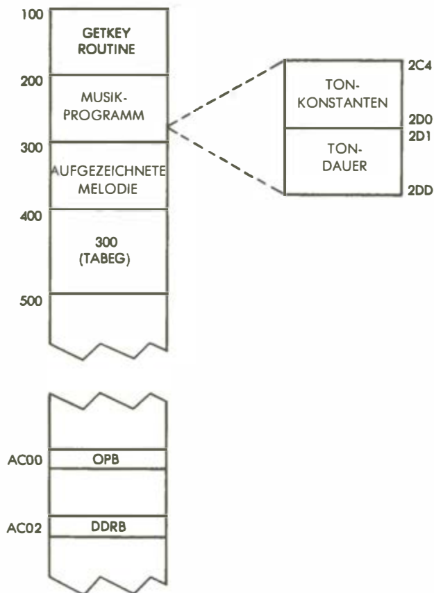
Abb. 2.4: Speicheraufteilung
