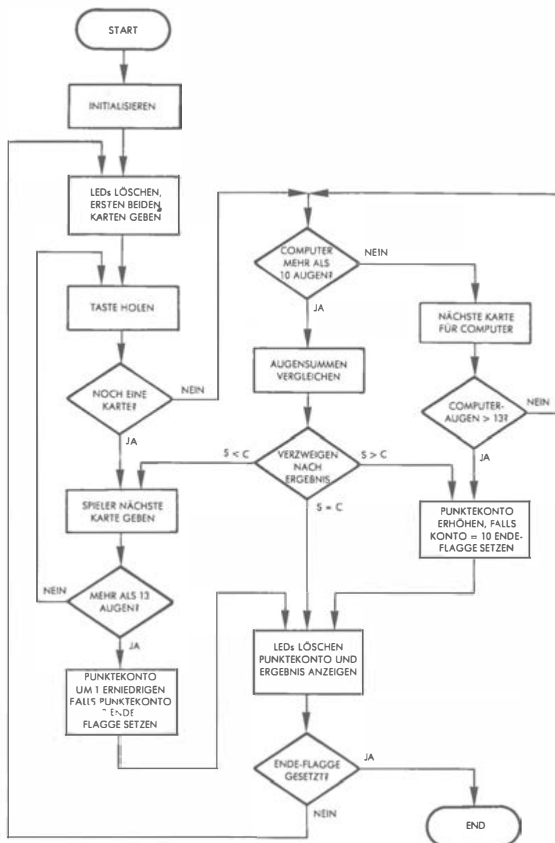
Abb. 10.9: Flußdiagramm „17+4“
