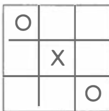
Abb. 11.41: Die Diagonalfalle
