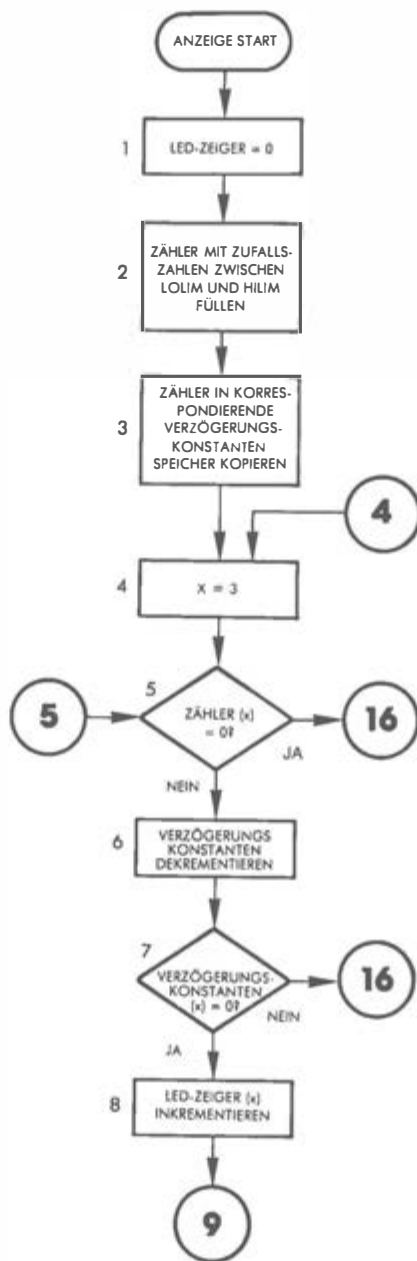
Abb. 7.4: Flußdiagramm DISPLAY
