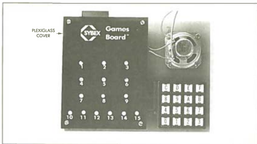
Abb. 1.18: „Produktions“-Spielbrett
