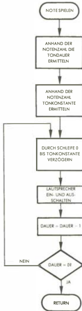
Abb. 2.8: Flußdiagramm PLAYIT
