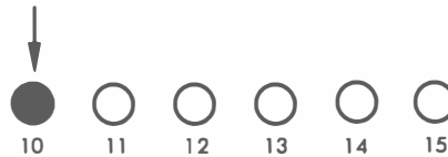
Abb. 9.1: Sequenzlänge eingeben
