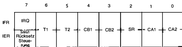
Bild 2.28: Die Interrupt-Register (IFR/IER)
