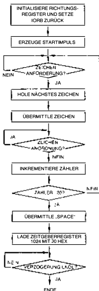
Bild 6.20: Flußdiagramm für Druckerprogramm
