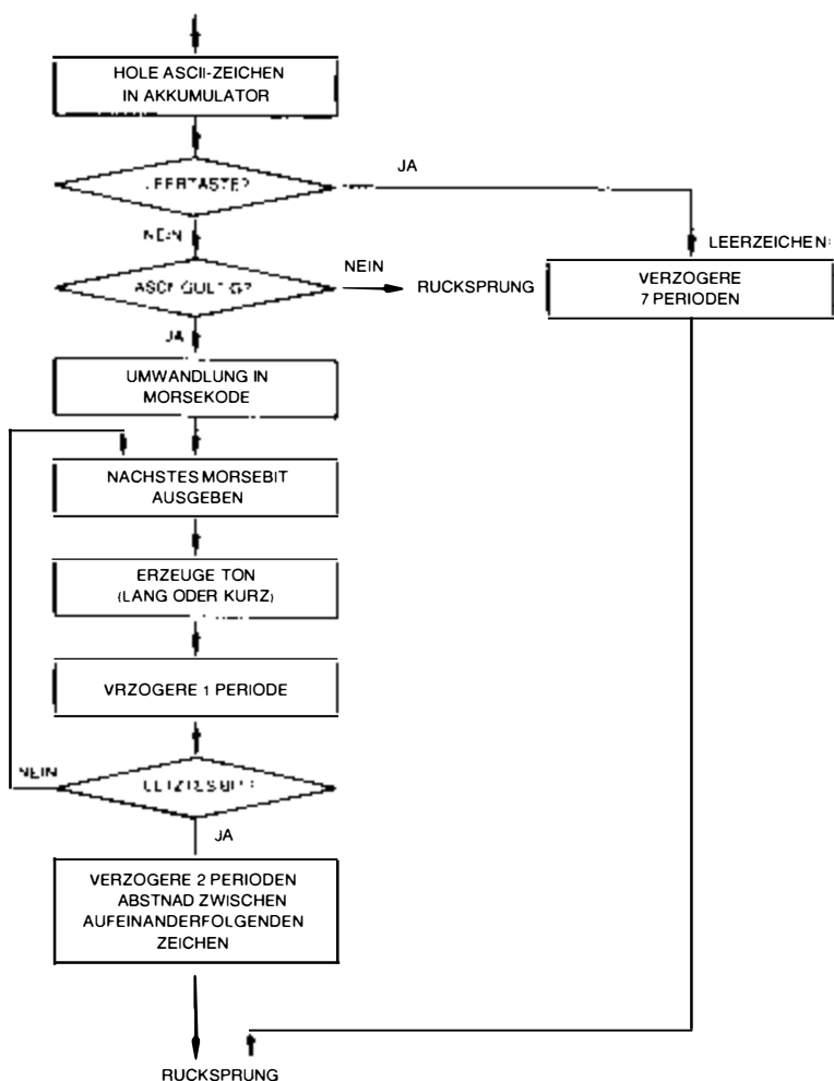
Bild 4.19: Flußdiagramm der Morsezeichenerzeugung
