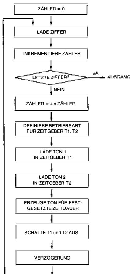
Bild 4.40: Telefonwähler, Flußdiagramm
