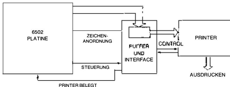
Bild 6.18: Standard-Druckerinterface
