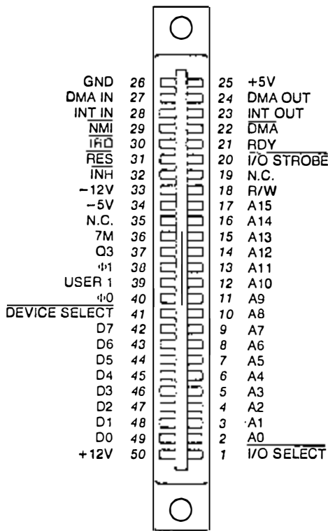
Bild 3.29: Periphere Ein/Ausgabestecker bei APPLE II (slots), Kontaktbelegung
