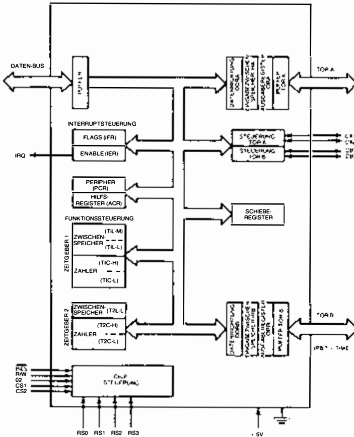
Bild 2.14: 6522interne Architektur
