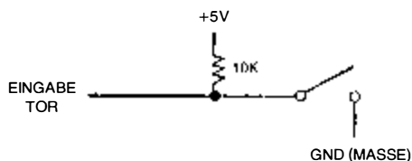
Bild 4.11: Anschluß eines Umschalters
