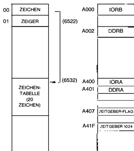
Bild 6.21: Druckerprogramm, Speicherbelegung
