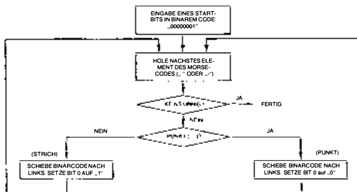
Bild 4.20: Umwandlung Morse nach binär
