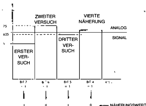
Bild 5.45: Sukzessive Approximation
