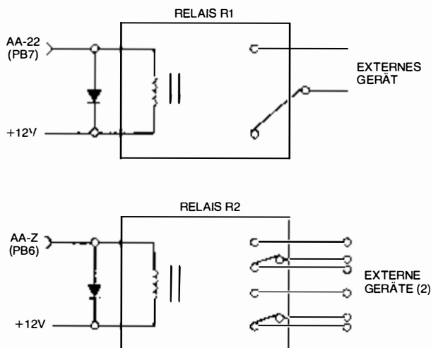
Bild 4.6: Anschluß zweier Relais an den PIO
