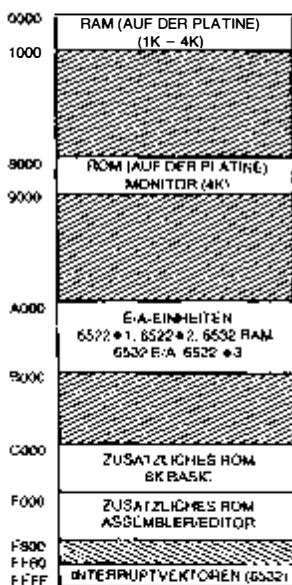
Bild 3.9: System-Speicheraufteilung
