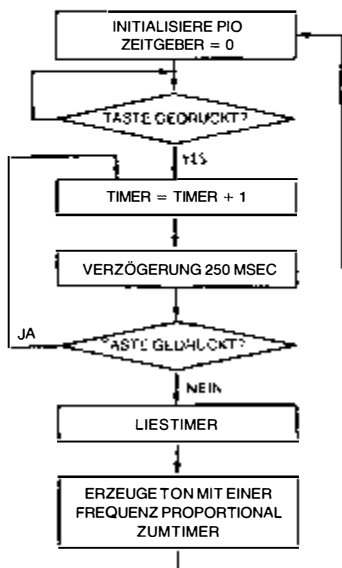
Bild 4.54: Programm zur Impulszeitmessung (Flußdiagramm)
