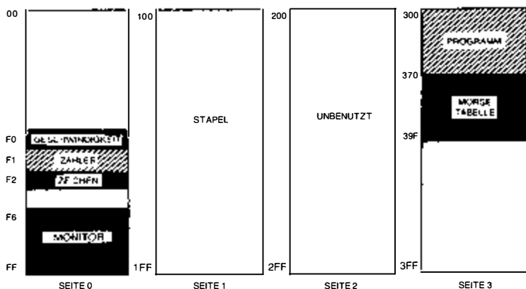
Bild 4.18: Speicherbelegung für das Morseprogramm
