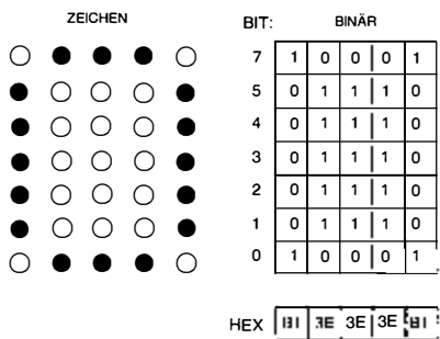
Bild 5.18: Anzeige einer „0“
