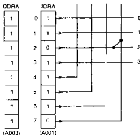
Bild 6.4: Vierter Schritt – IORA wieder einlesen
