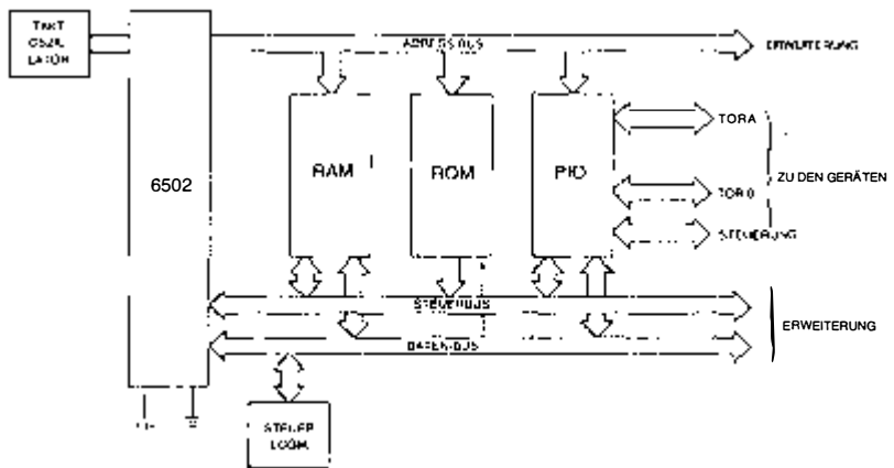
Bild 3.1: Organisation eines „Standard“-6502-Systems
