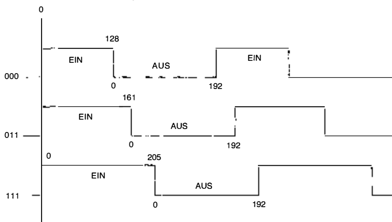
Bild 5.42: Die Formen des Ausgangssignals
