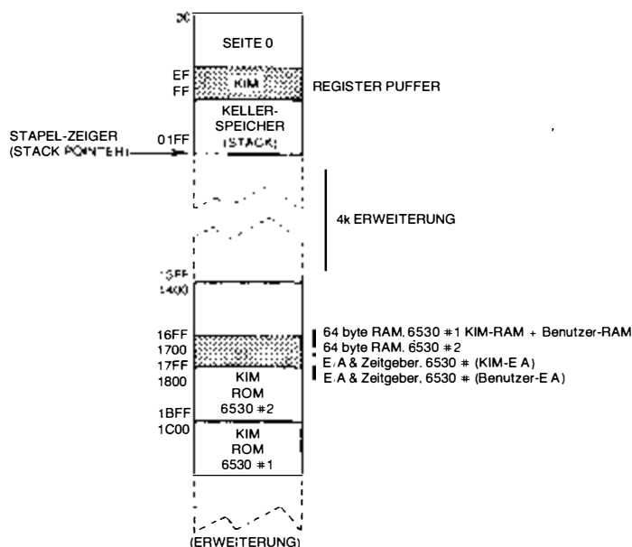
Bild 3.4: KIM-1 Speicheraufteilung
