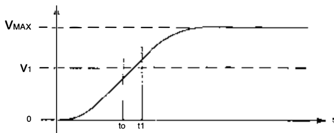
Bild 5.39: Geschwindigkeitskurve des Gleichstrommotors
