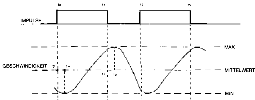
Bild 5.37: Digitale Drehzahlsteuerung
