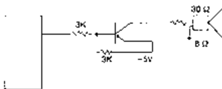
Bild 4.50: Verbesserter Anschluß eines Lautsprechers
