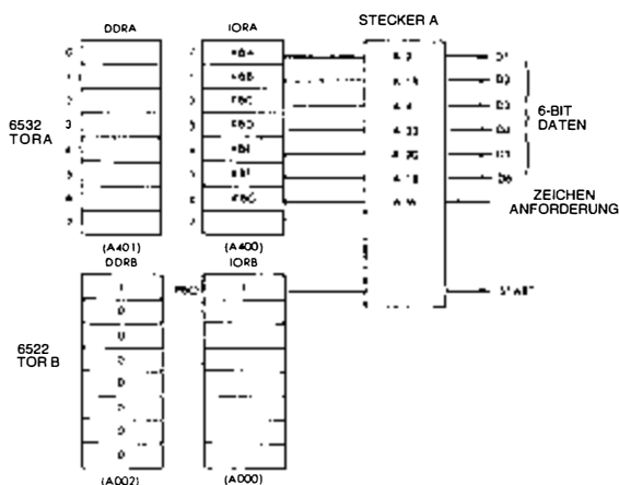
Bild 6.19: Anschluß des Druckers
