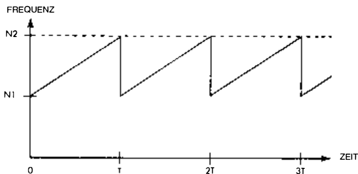
Bild 5.34: Ein Sirenenton
