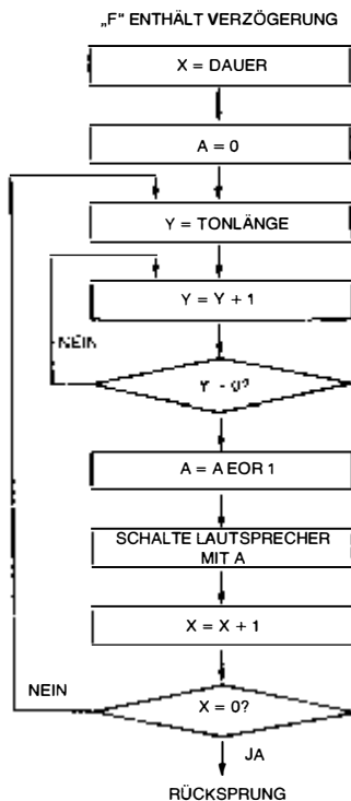
Bild 4.63: Flußdiagramm zum Musikprogramm
