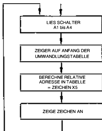
Bild 5.23: Anzeige von Schalterstellungen
