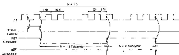
Bild 2.32: Zeitgeber 1 im Freilaufmodus
