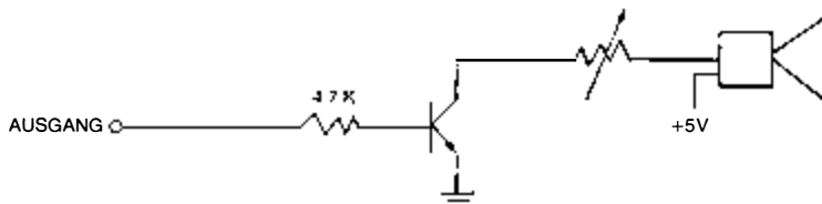
Bild 4.17: Erzielen eines lauterer Tones
