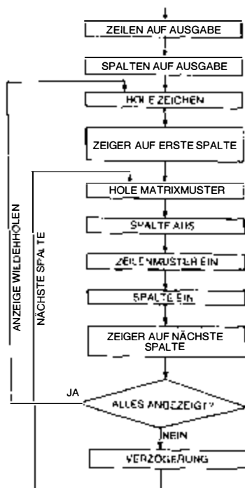
Bild 5.20: Treiberprogramm für eine Punktmatrix aus LED's
