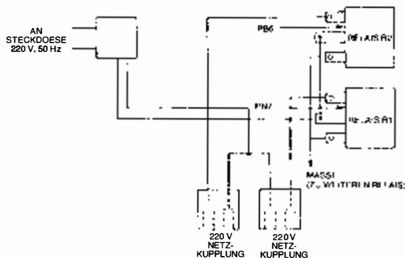
Bild 4.7: Externe Beschaltung der Relais
