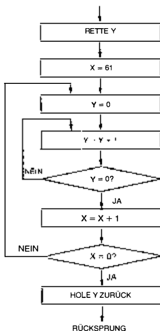
Bild 4.56: 250msec Verzögerung, Flußdiagramm
