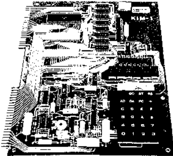
Bild 3.2: Der KIM-1
