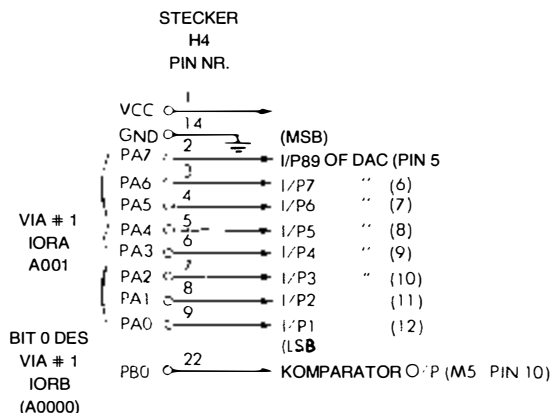
Bild 5.48: Anschluß an Stecker H4
