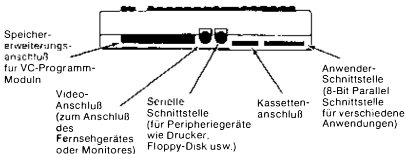
Bild 3.25: Rückansicht des VC-20, schematisch
