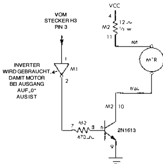
Bild 5.36: Anschluß des Motors
