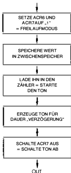
Bild 4.28: Erzeugen eines Tones bestimmter Dauer mit Zeitgeber 1
