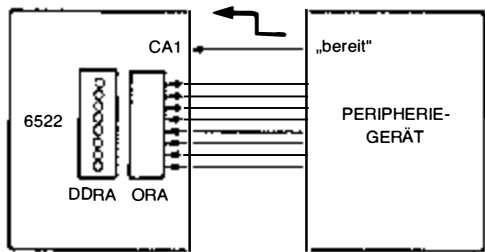
Bild 2.26: Einlesen von Daten im Bereit-Zustand des Gerätes
