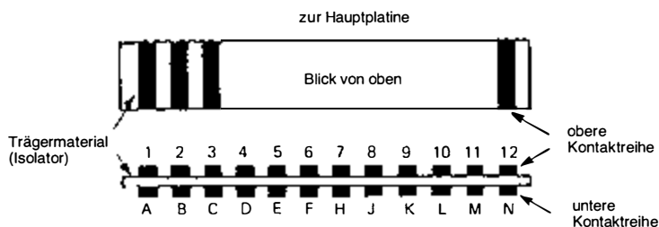
Bild 3.21: Blick auf den USER-port und Kontaktbenennung
