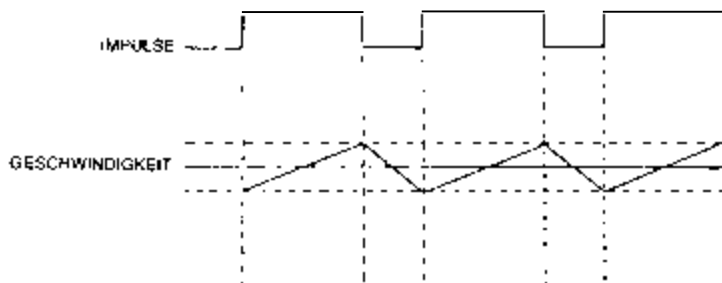
Bild 5.38: Vereinfachtes Geschwindigkeitsdiagramm
