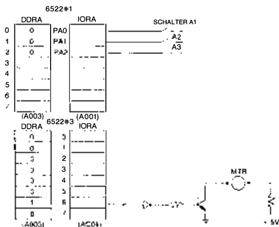
Bild 5.40: Das Anschlußbild
