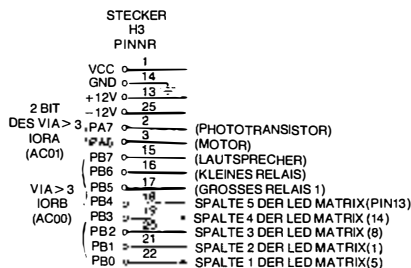
Bild 5.17b: Anschluß der LED's (Spalten)
