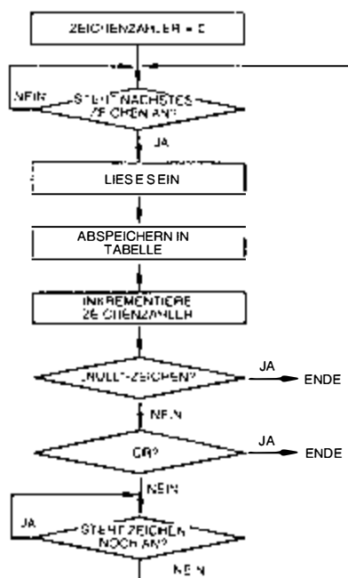
Bild 6.14: Programm Lochstreifenleser, Flußdiagramm
