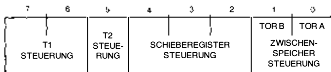
Bild 2.27: Hilfs-Steuerregister (ACR)
