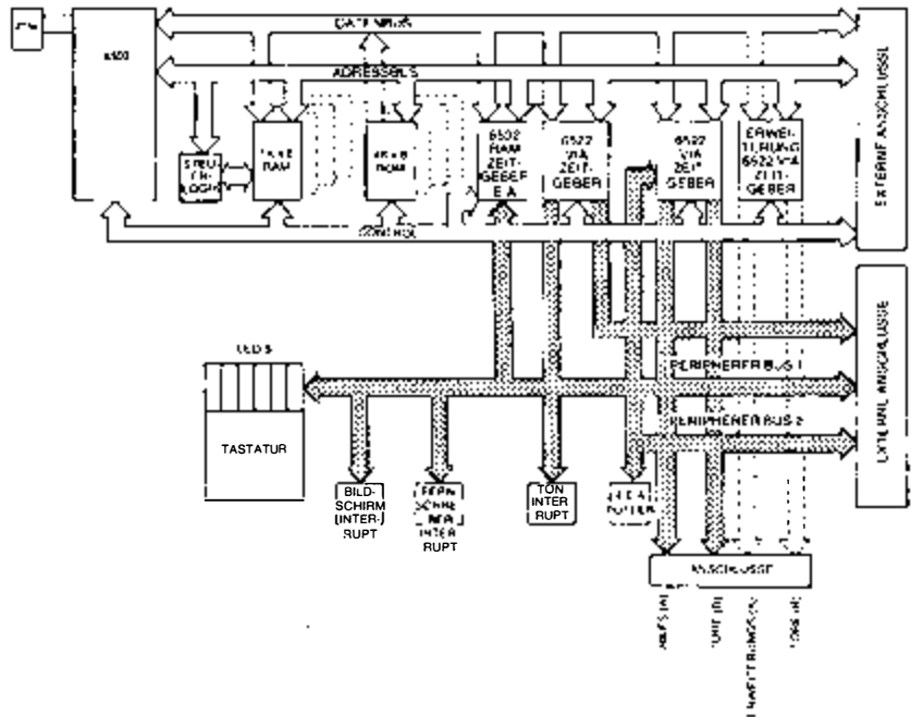
Bild 3.8: Interne Organisation des SYM
