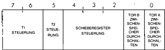
Bild 4.25: 6522 Hilfssteuerregister ACR
