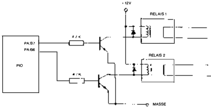
Bild 4.2: Relais-Interface
