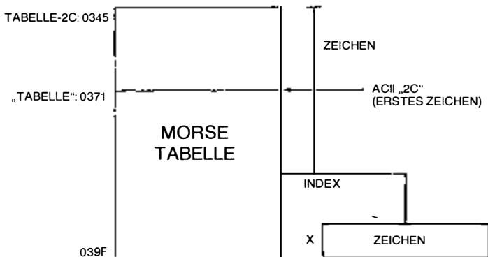
Bild4.32: Verwendung indizierter Adressierung zur Dekodierung des binären Morse-Kodes
