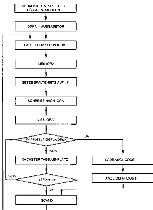
Bild 6.6: Tastatur-Programm, Flußdiagramm
