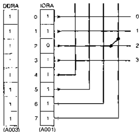
Bild 6.3: Dritter Schritt – Schreiben in IORA
