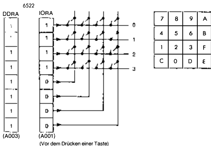
Bild 6.1: Anschluß der Tastatur
