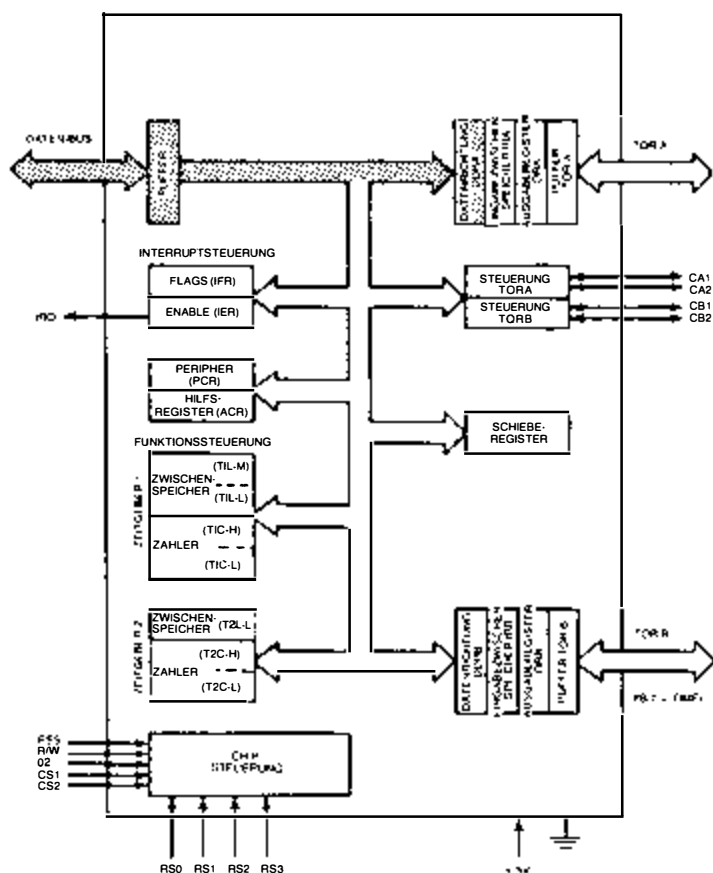
Bild 2.17: Gebrauch des 6522: STA DDRA
