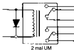
Bild 4.5: Anschluß eines Relais mit 2 Kontakten
