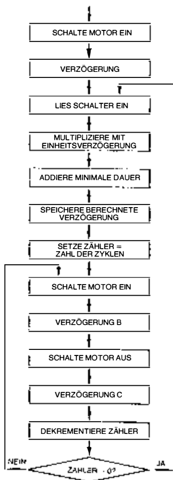
Bild 5.41: Gleichstrommotor, Flußdiagramm
