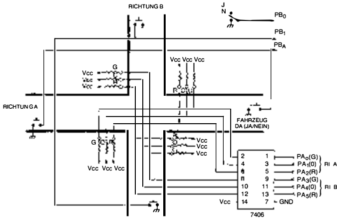
Bild 4.66: Verdrahtung der simulierten Ampelanlage
