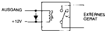
Bild 4.3: Anschluß eines einfachen Relais (Arbeitskontakt)
