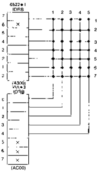
Bild 5.16: Anschluß der 5 x 7 LED-Matrix
