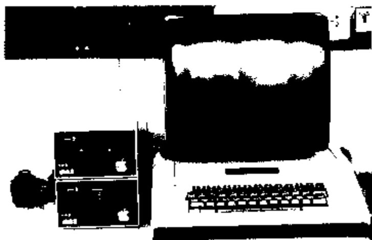
Bild 3.27: APPLE II mit Monitor und zwei Diskettenlaufwerken
