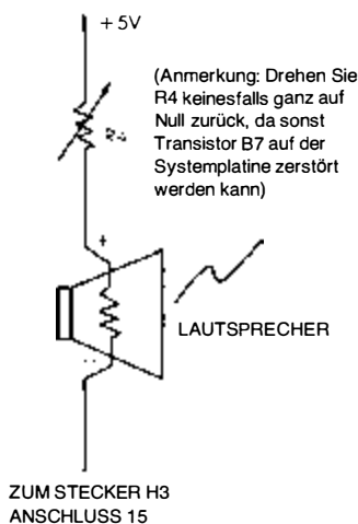
Bild 5.25: Anschluß des Lautsprechers
