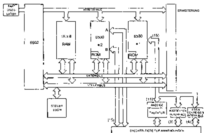
Bild 3.3: Interne Organisation des KIM-1
