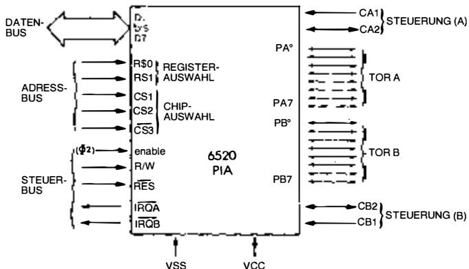
Bild 2.2: Der 6520 PIA
