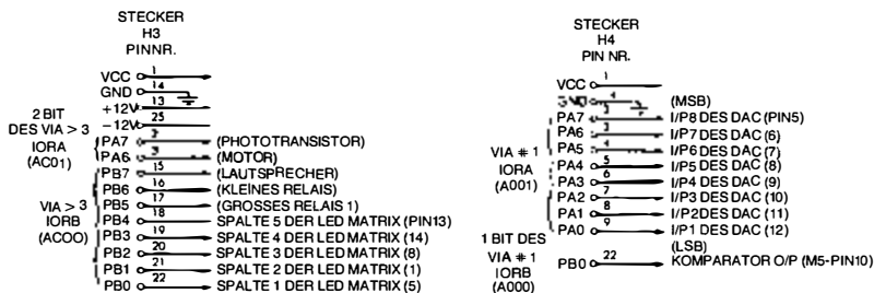
Bild 5.5B: Die Stecker H3 und H4
