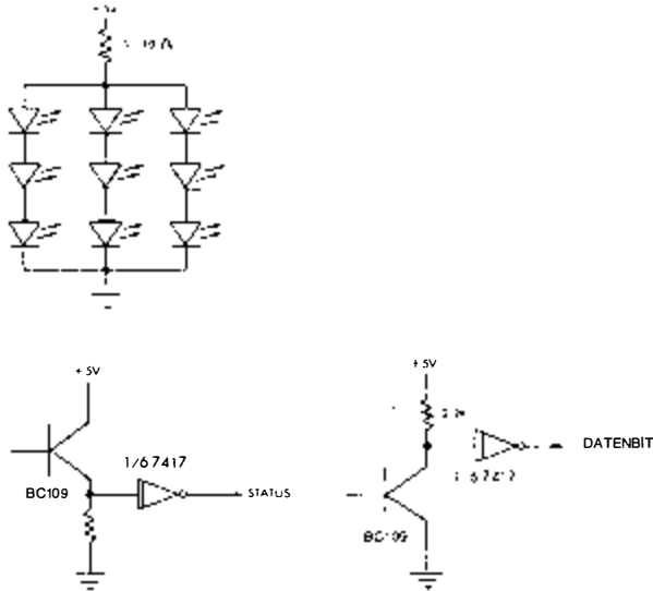
Bild 6.12: Lochstreifenleser, Anschlußdetails
