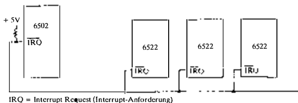
Bild 2.35: Anschluß mehrerer 6522: Interrupt-Anforderung
