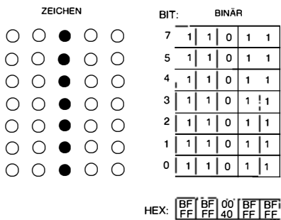
Bild 5.19: Anzeige einer „1“
