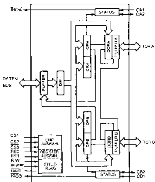
Bild 2.3: 6520, interne Architektur
