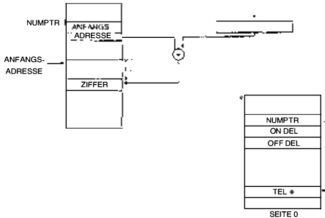
Bild 4.42: Telefonwähler: Indirekt indizierter Zugriff (oben) und Speicherbelegung (unten)
