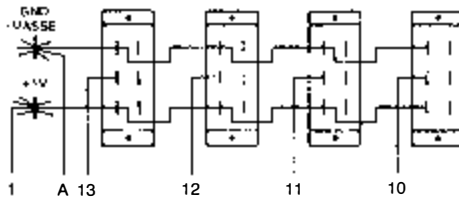
Bild 4.15: Anschlußdetails bei vier Umschaltern
