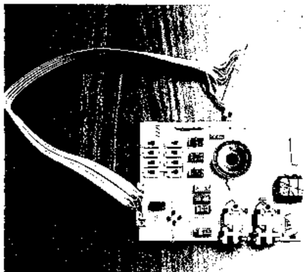
Bild 5.3: Bequemer Anschluß der Benutzerplatine an den Computer mit Steckverbindungen
