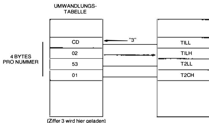
Bild 4.43: Laden des Zeitgebers
