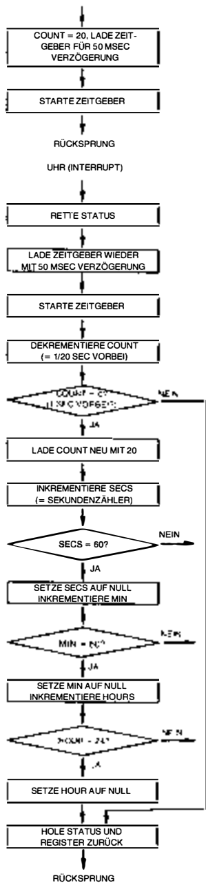
Bild 4.36: 24-Stunden-Uhr, Flußdiagramm
