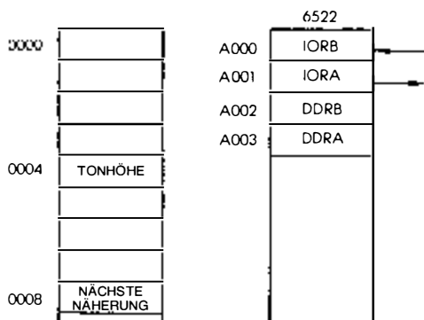
Bild 5.49: Speicherbelegung des A/D-Wandlers
