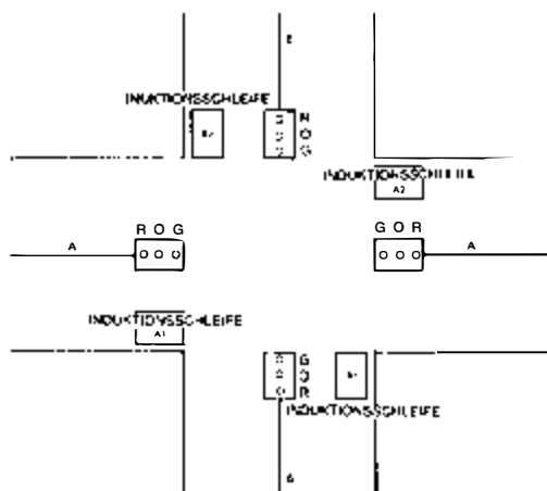
Bild 5.6: Das Verkehrssteuersystem
