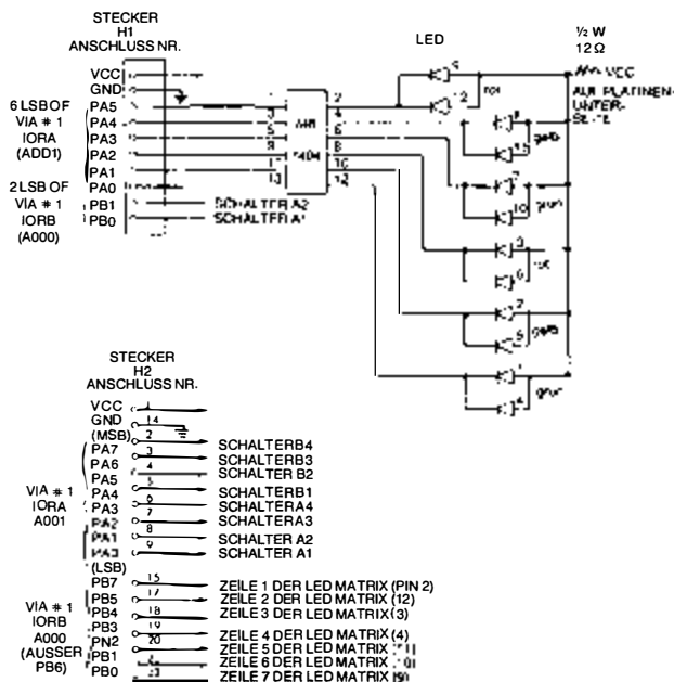
Bild 5.5A: Stecker H1 und H2
