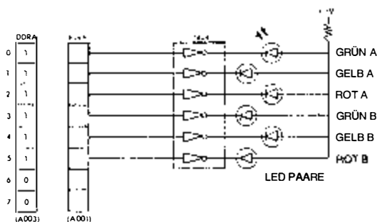
Bild 5.7: Anschluß der LED's
