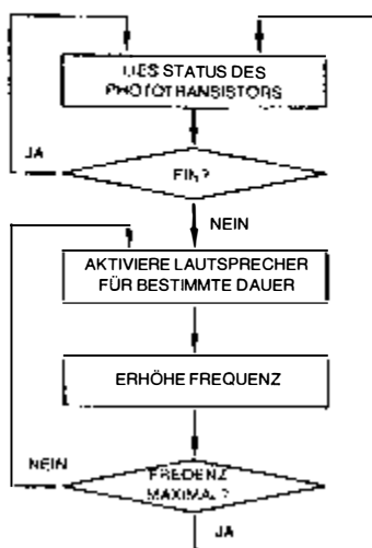
Bild 5.33: Alarmanlage, Flußdiagramm
