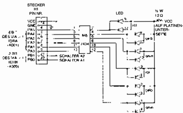
Bild 5.8: Verdrahtung aller LED's
