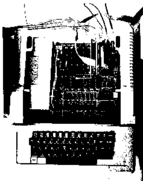
Bild 3.28: APPLE II, Blick in Gehäuseinneres
