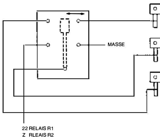
Bild 4.10: Detail des Relaisanschlusses an die Anwenderplatine
