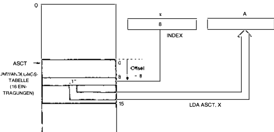
Bild 6.9: Umwandlung des IORA-Kodes in ASCII
