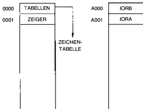
Bild 6.15: Lochstreifenleser, Speicherbelegung
