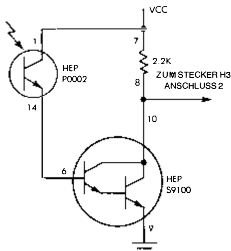
Bild 5.32: Die Schaltung des Phototransistors (auf Sockel M3)
