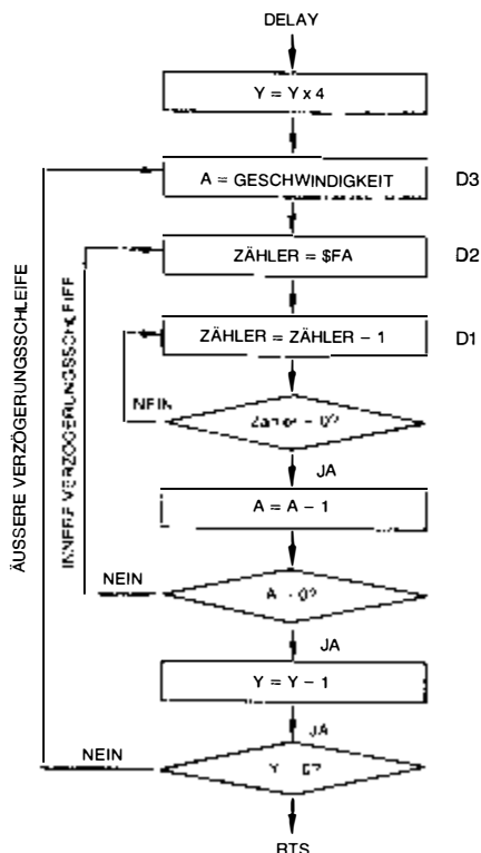
Bild 4.34: Flußdiagramm des Unterprogramms DELAY
