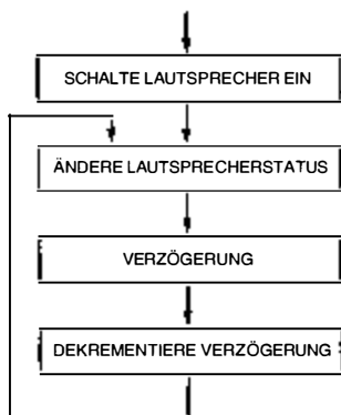
Bild 4.47: Flußdiagramm „Sirene“ – positive Rampe
