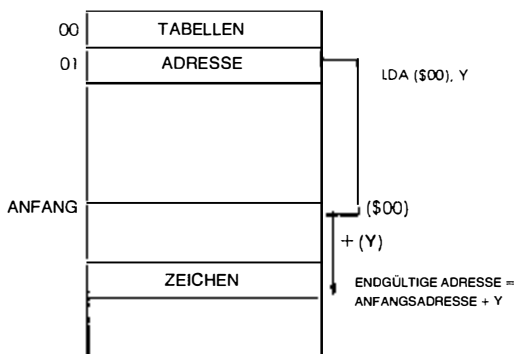
Bild 6.23: Indirekt indizierte Adressierung
