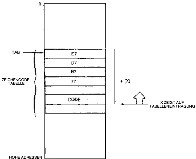
Bild 6.8: Tabellenzugriff durch indizierte Adressierung
