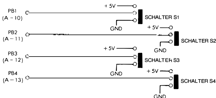
Bild 4.13: Anschluß von vier Umschaltern an den SYM
