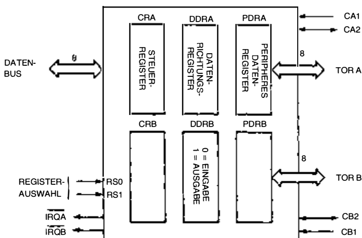
Bild 2.1: Typischer PIO
