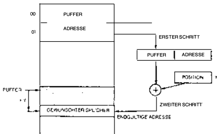
Bild 6.17: Indirekt indizierter Zugriff: STA ($00),Y
