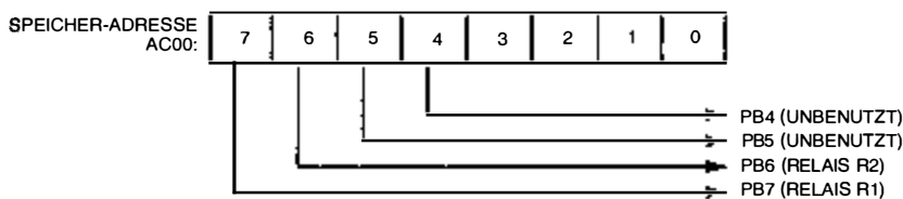
Bild 4.9: Tor B des 6522 #3
