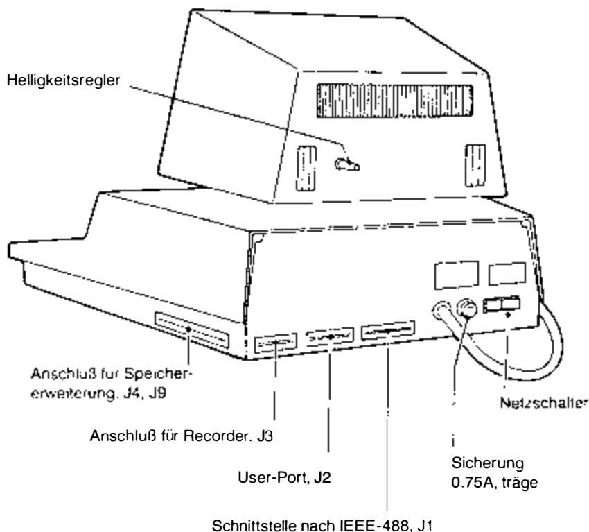
Bild 3.20: Rückseite des CBM 4032
