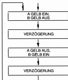
Bild 5.9: Nachtsteuerung
