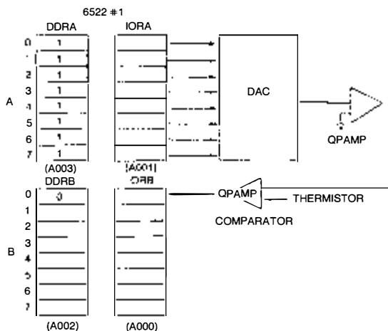
Bild 5.44: Anschluß zur Analog-Digital-Wandlung
