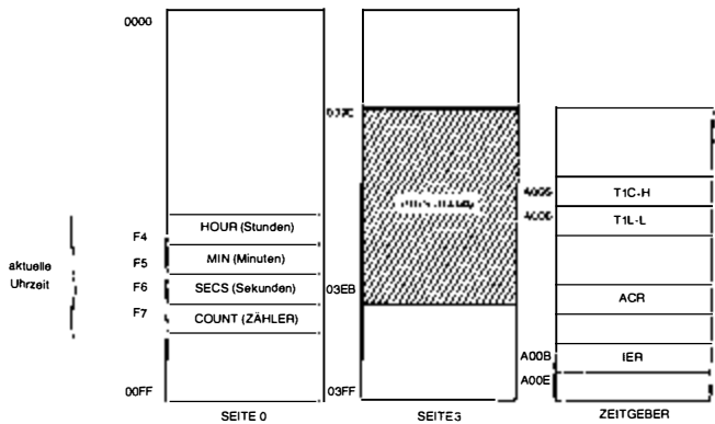
Bild 4.35: 24-Stunden-Uhr, Speicherbelegung
