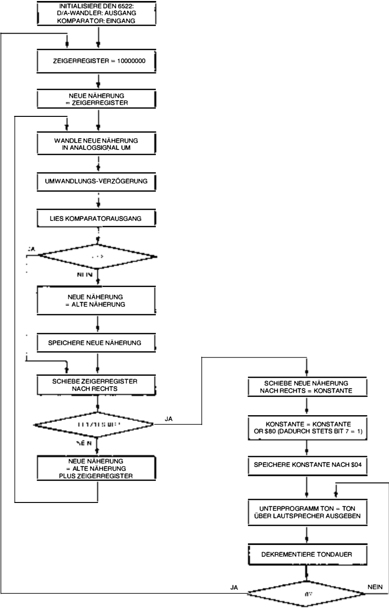
Bild 5.50: Flußdiagramm des Programms A/D-Wandlung
