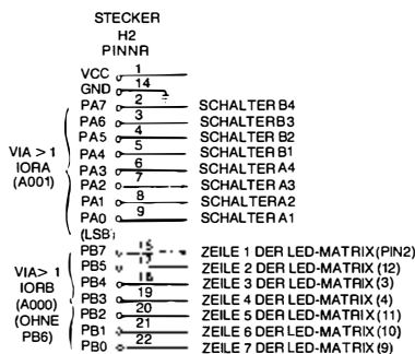
Bild 5.17a: Anschluß der LED's (Zeilen)
