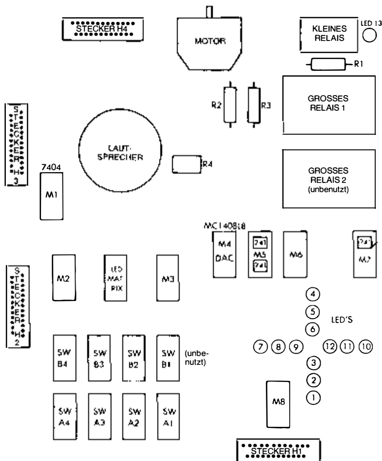
Bild 5.4: Anordnung der Bauteile auf der Platine
