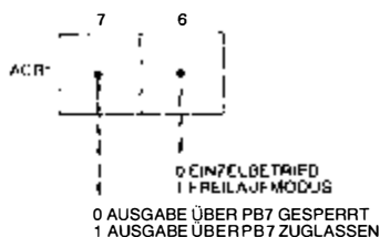
Bild 2.29: 6522: Hilfs-Steuerregister steuert Betriebszustände von Zeitgeber 1 (T1)
