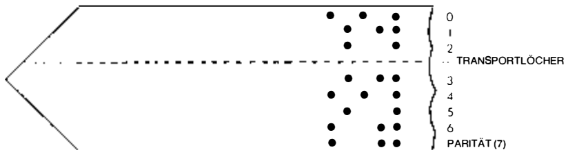
Bild 6.10: Ein 8-Bit Lochstreifen
