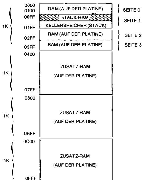
Bild 3.10: RAM-Speicheraufteilung
