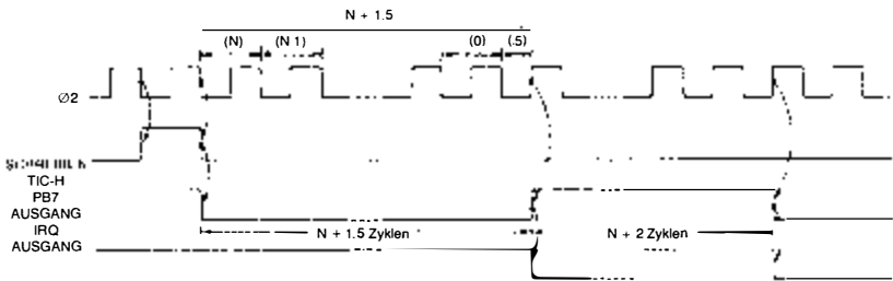
Bild 4.26: Diagramm der zeitlichen Abfolge bei der Tonerzeugung
