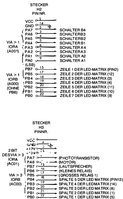
Bild 5.31: Verbindungen für das Musikprogramm
