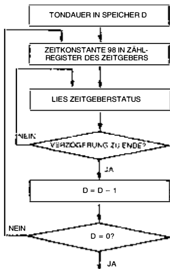
Bild 4.58: Flußdiagramm der Routine TIME10 (erzeugt Verzögerung von 0,1 sec)
