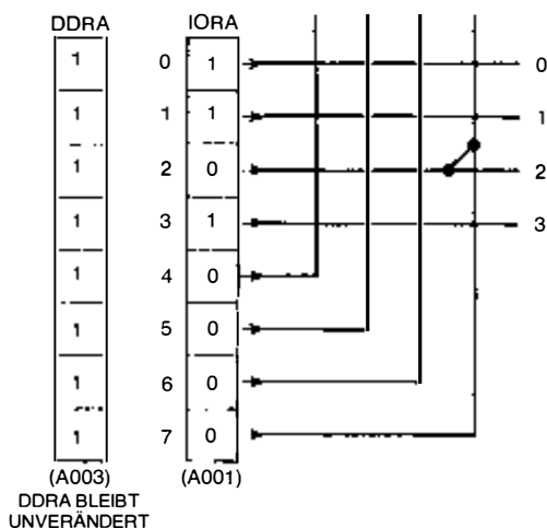
Bild 6.2: Zweiter Schritt – Lesen des IORA nach Schließen des Tastenkontaktes
