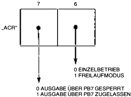
Bild 4.30: Die Bits 6 und 7 des ACR
