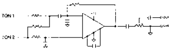
Bild 4.45: Vorschlag für hardwareseitige Verbesserung für sauberere Frequenzen
