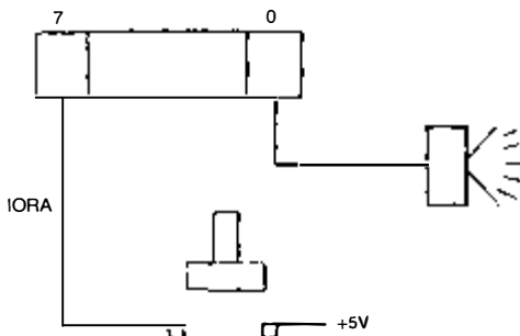
Bild 4.51: Anschluß des Lautsprechers und des Tasters
